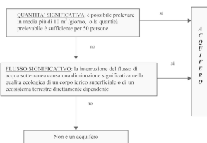
Figura 1: schema per l'identificazione degli acquiferi
