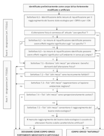
Fig. 3 - Fasi del livello 2 per la designazione dei corpi idrici fortemente modificati e artificiali
