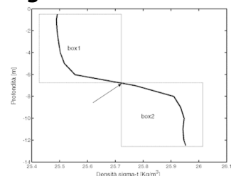
Figura 3.1 Relazione tra profondità e densità
